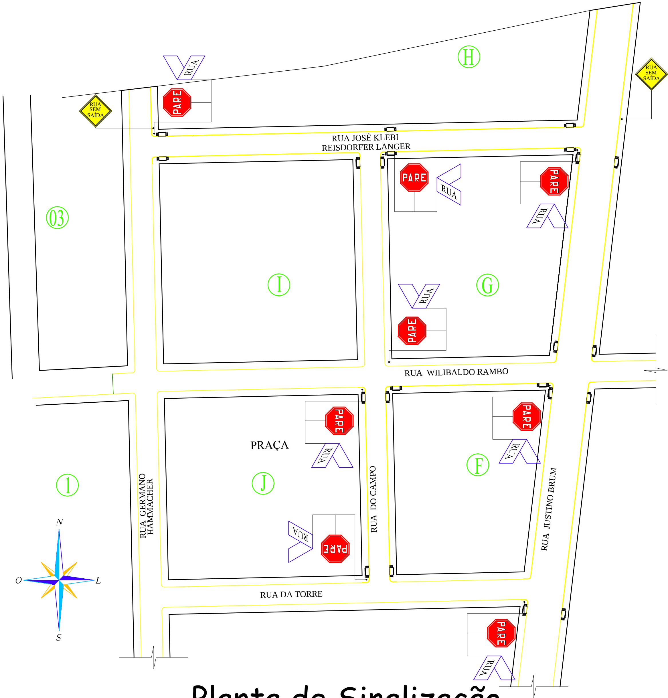
Planta de Sinalização Escala 1:750
